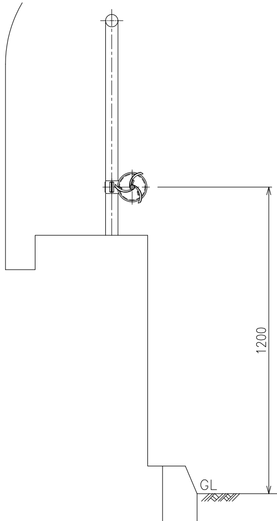
設置図 S=1:15
